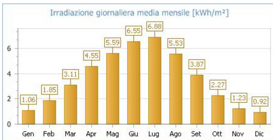
Fig. 2: Irradiazione giornaliera media mensile sul piano orizzontale [kWh/m²]- Fonte dati: UNI 10349 - Località di riferimento: CREMONA (CR)/MANTOVA (MN)
