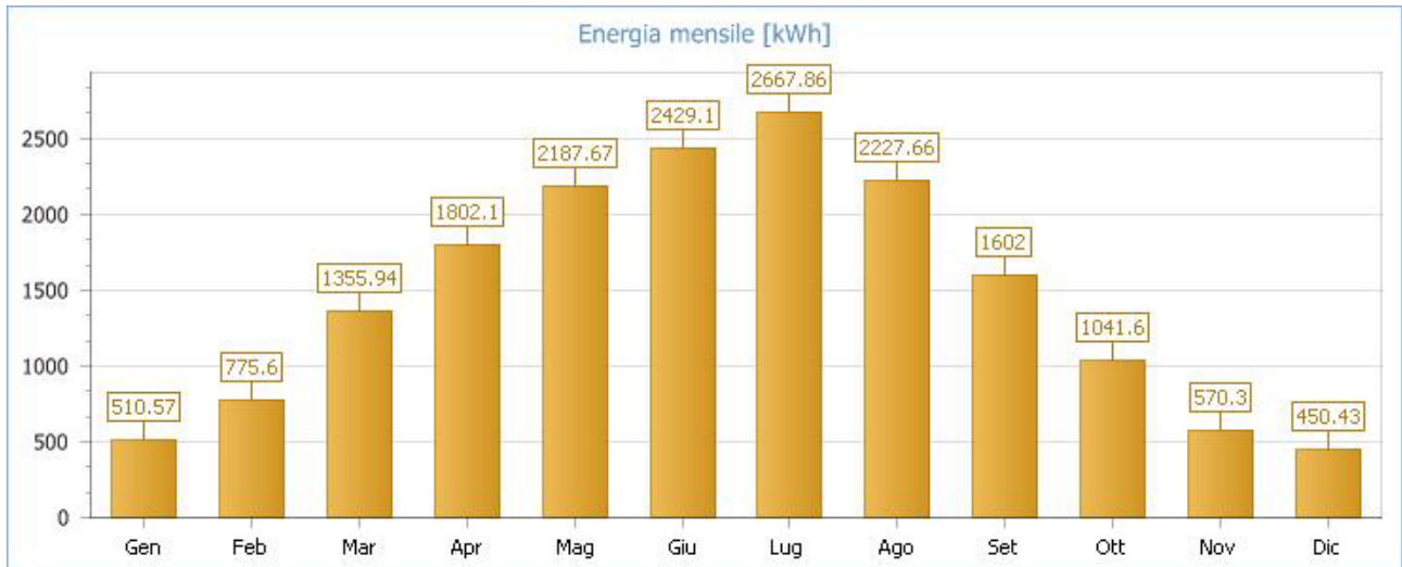
Fig. 4: Energia mensile prodotta dall'impianto
